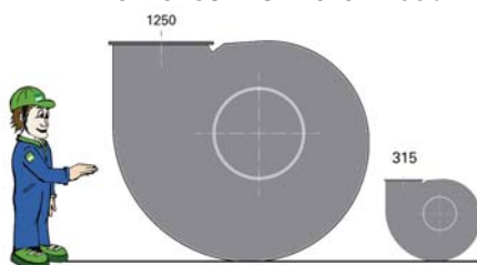
Fläktar CHVN 315 - 1250
